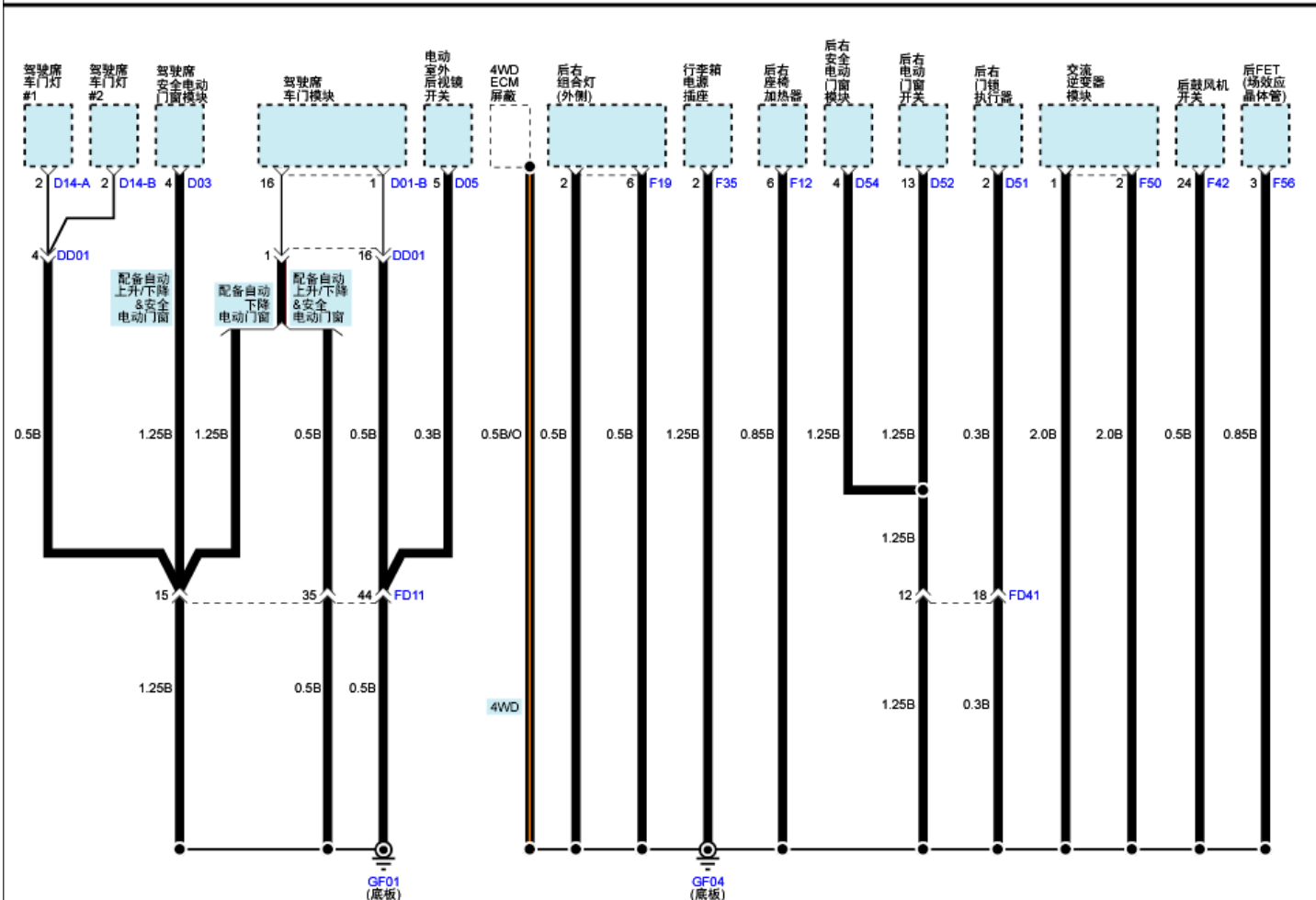
搭铁分布(12)
